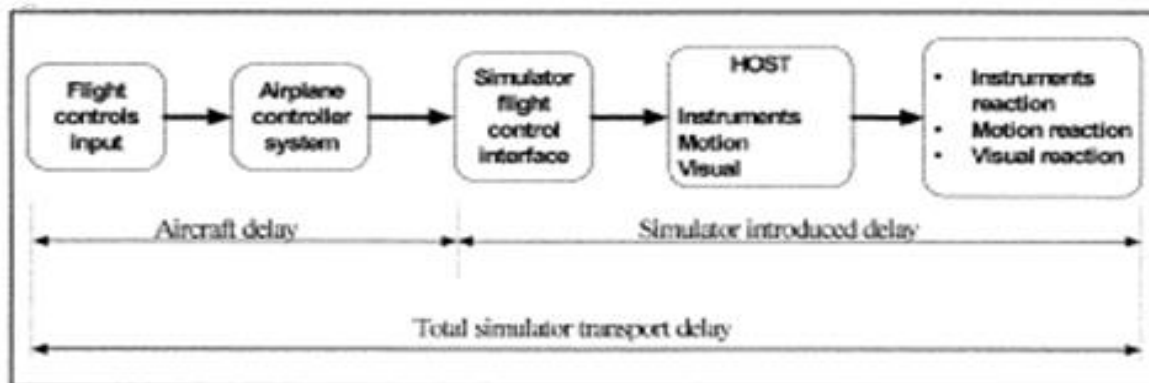
Figura A2D – Retardo para la simulación de aeronaves controladas por computadoras usando equipamiento real de la aeronave emulada (cajas negras)
