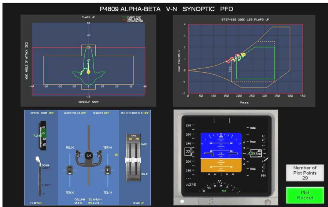
Figura 2 – Ejemplo de presentación UPRT en la pantalla de la IOS.
