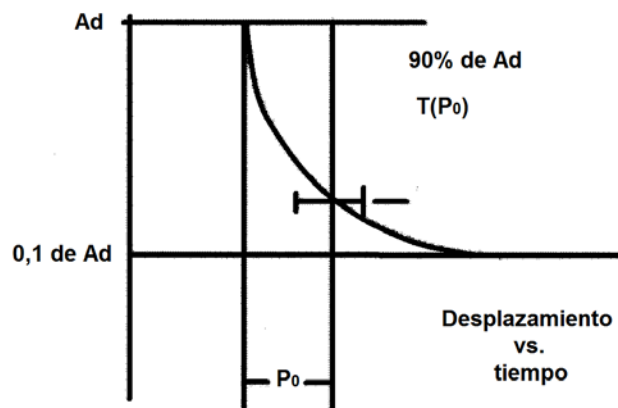
Figura D2B – Respuesta con amortiguación crítica
