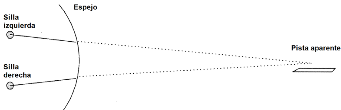
Figura C2J – Visualización de la pista en una pantalla colimada
