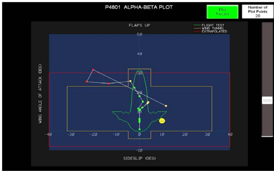
Figura 1 – Ejemplo de diagrama de una envolvente Alfa/Beta.
