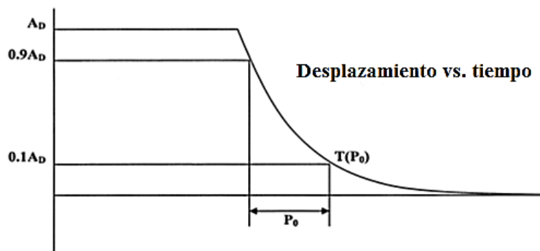
Figura C2B – Respuesta al movimiento momentáneo de un sistema crítico o de alta amortiguación.
