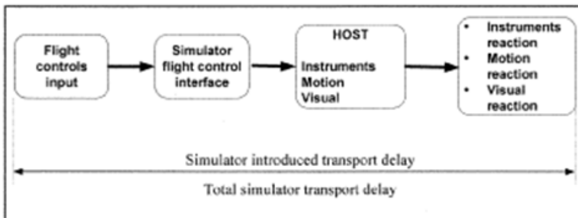
Figura A2C – Retardo para la simulación de aviones que no son controlados por computador
