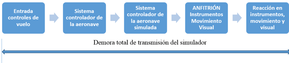
Figura C2G – Tiempos de transmisión para simulación de aeronaves controladas por computador usando emulación de software de cajas negras de helicóptero
