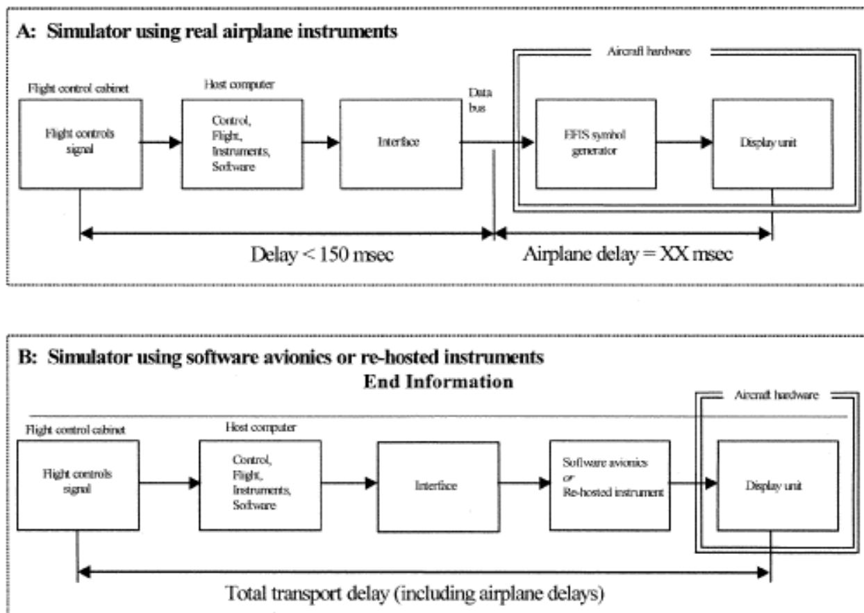
Figuras A2F(A) y A2F(B) – Retardo para la simulación de aeronaves usando instrumentos reales o integrados de la aeronave emulada
