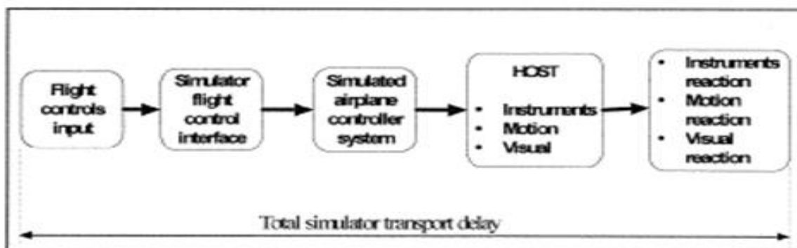
Figura A2E – Retardo para la simulación de aeronaves controladas por computadoras usando equipamiento simulado de la aeronave emulada
